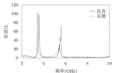
图6 天线驻波比实测与仿真对比图
