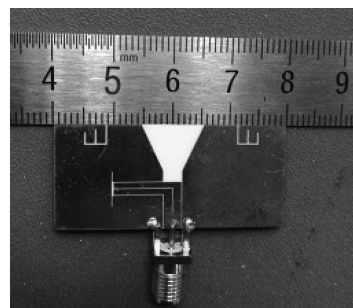
图5 天线实物图
