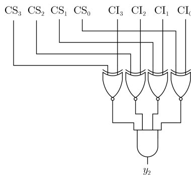
图7 密钥确认模块 [14]
