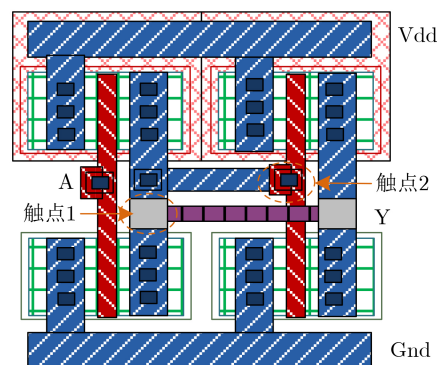
图1 INV/BUF伪装单元结构 [14]
