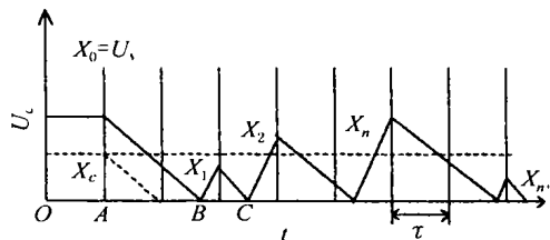
图 2 电容电压变化图
