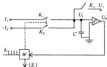
图 1 测量电路
