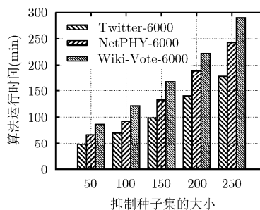
图7 SAA-mining 算法的运行时间图
