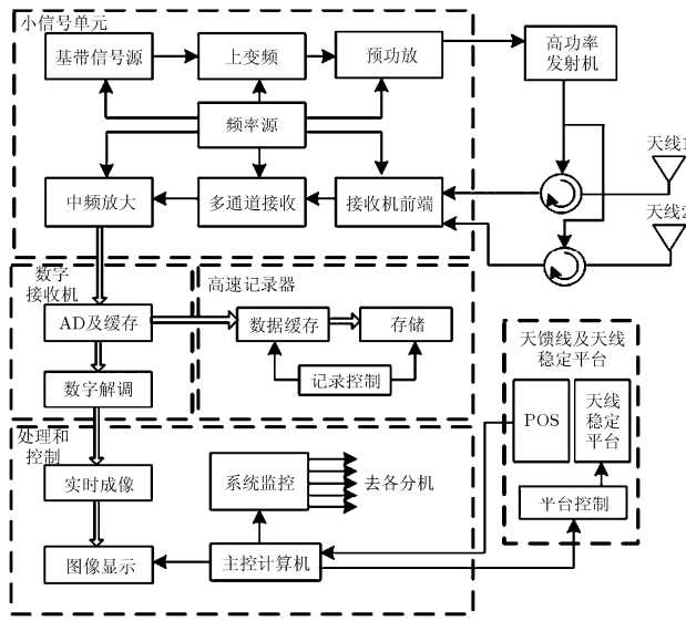
图 2 系统组成框图
