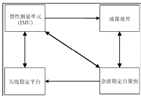
图10 高分辨率 SAR 系统运动补偿方案
