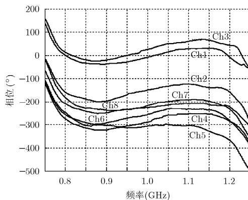
图5 雷达接收机相位特性曲线
