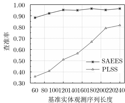
图7 不同基准实体观测序列长度下的查准率
