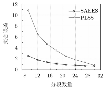
图2 不同分段数量下的拟合误差
