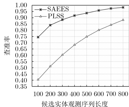
图6 不同候选实体观测序列长度下的查准率
