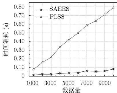
图3 不同数据量下的分段时间消耗
