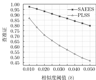
图4 不同相似度阈值下传感器的查准率
