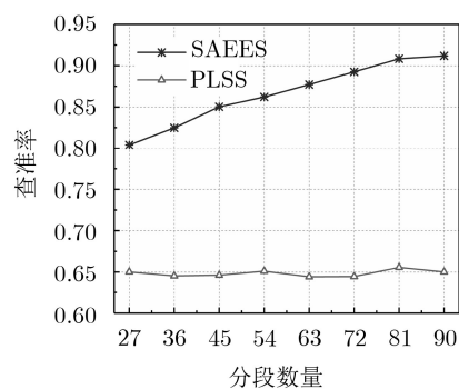
图5 不同分段数下的查准率
