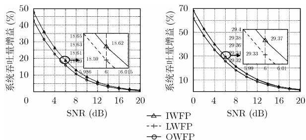
图1 \text{BER} = 10^{-3} 时系统
