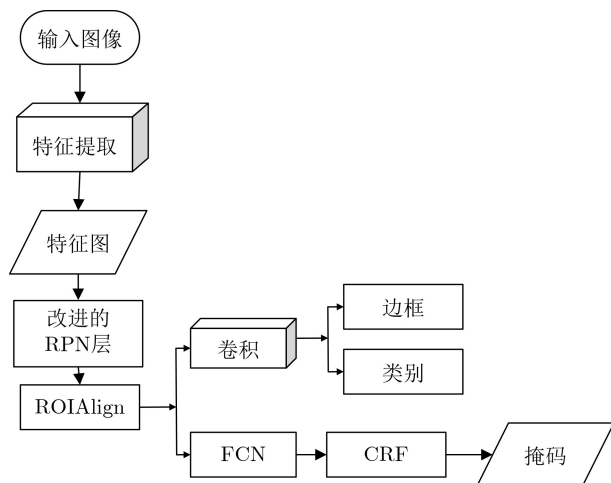
图2 改进后Mask R-CNN流程图
