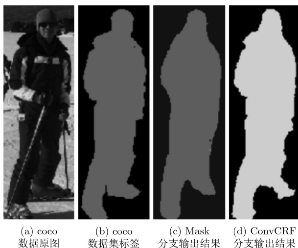
图4 改进的Mask分支和原分支输出图像对比
