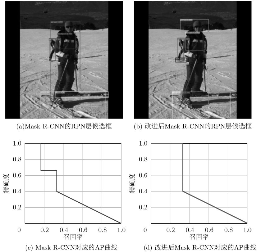
图 5 RPN层可视化结果
