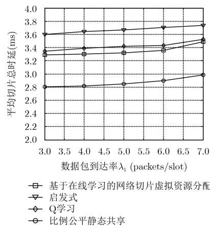
图5 不同数据包到达率 \lambda_1 下的平均切片总时延
