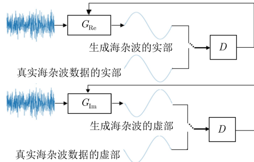
图2 海杂波数据对抗生成网络结构
