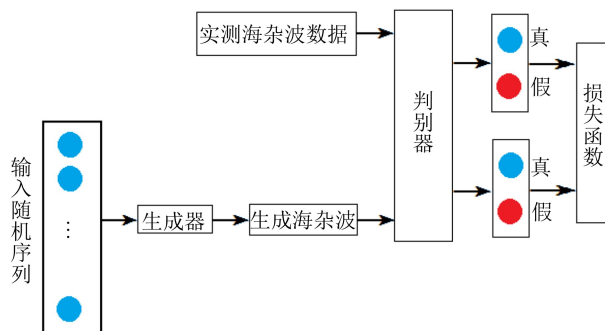
图1 GAN结构示意图
