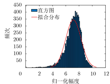
图8 第100采样点10000帧海杂波幅度直方图
