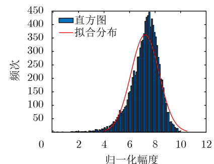
图9 生成海杂波数据(10000帧)幅度直方图
