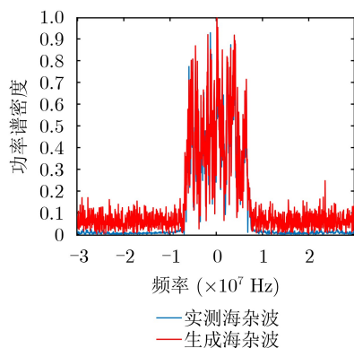
图12 实测海杂波数据&amp;生成海杂波数据功率谱密度
