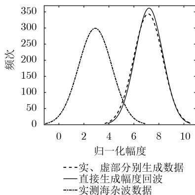
图11 幅度分布拟合曲线
