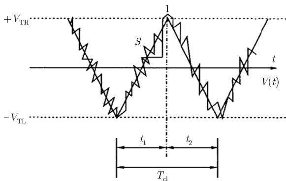
图3 带噪声的三角波
