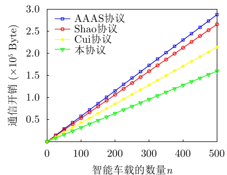
图3 RSU端通信开销对比
