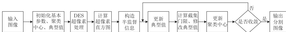
图1 desSS-C-PCM算法流程图
