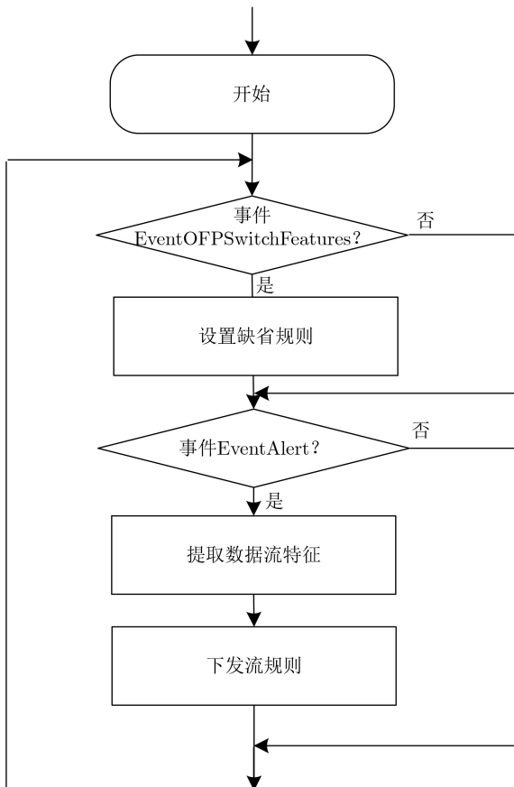
图5 转发处理模块处理过程
