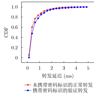
图7 转发延迟CDF
