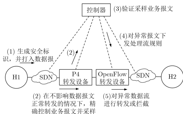
图3 转发验证过程
