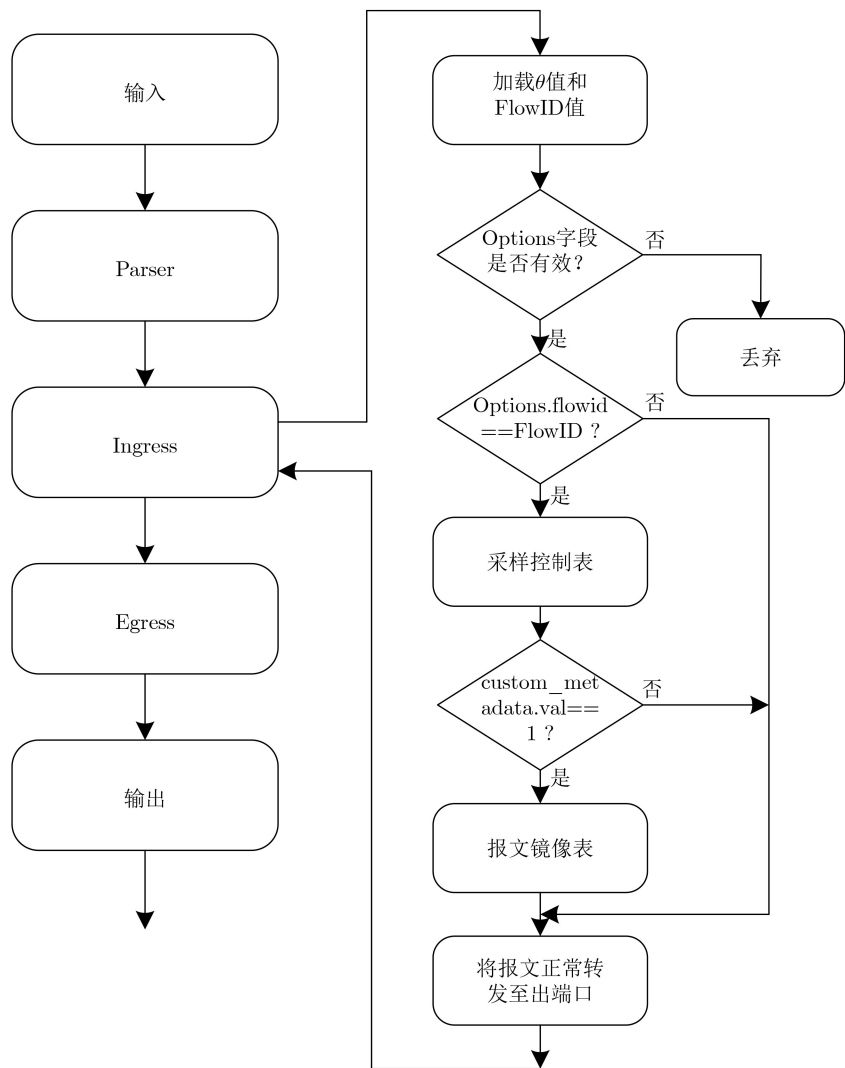
图4 控制程序流程图
