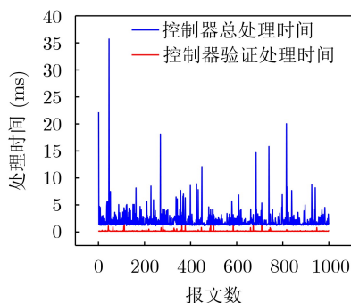
图9 控制器处理时间
