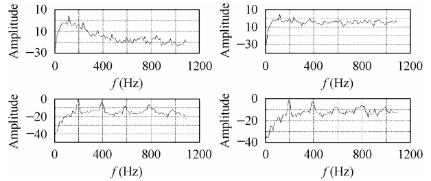
图3 谐波积谱法检测基音频率( r=1\sim5 ) (a)男声在无噪声时的对数谐波积谱 (b)男声在SNR=10dB时的对数谐波积谱 (c)女声在无噪声时的对数谐波积谱 (d)女声在SNR=10dB时的对数谐波积谱
