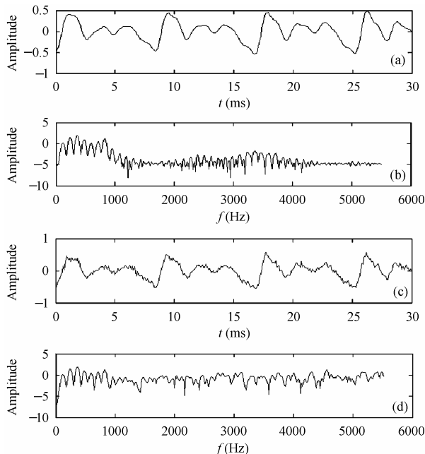
图 1 男声浊音帧的时域波形和短时谱 (a) 无噪声时的时域波形 (b) 无噪声时的对数谱 (c) SNR=10dB 时的时域波形 (d) SNR=10dB 时的对数谱
