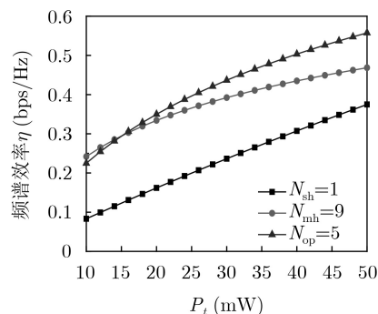
图5 \beta_T=40^\circ , \beta_R=20^\circ 的3种通信方式对比
