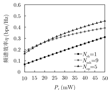
图4 \beta_T=\beta_R=30^\circ 的3种通信方式对比
