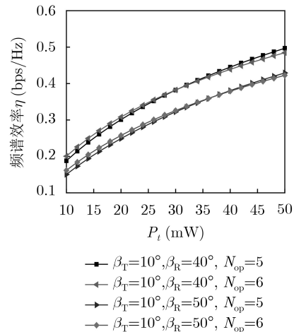
图8 两种方法传输能力对比
