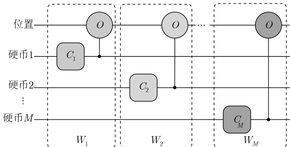
图1 基于多个硬币的量子游走线路原理图
