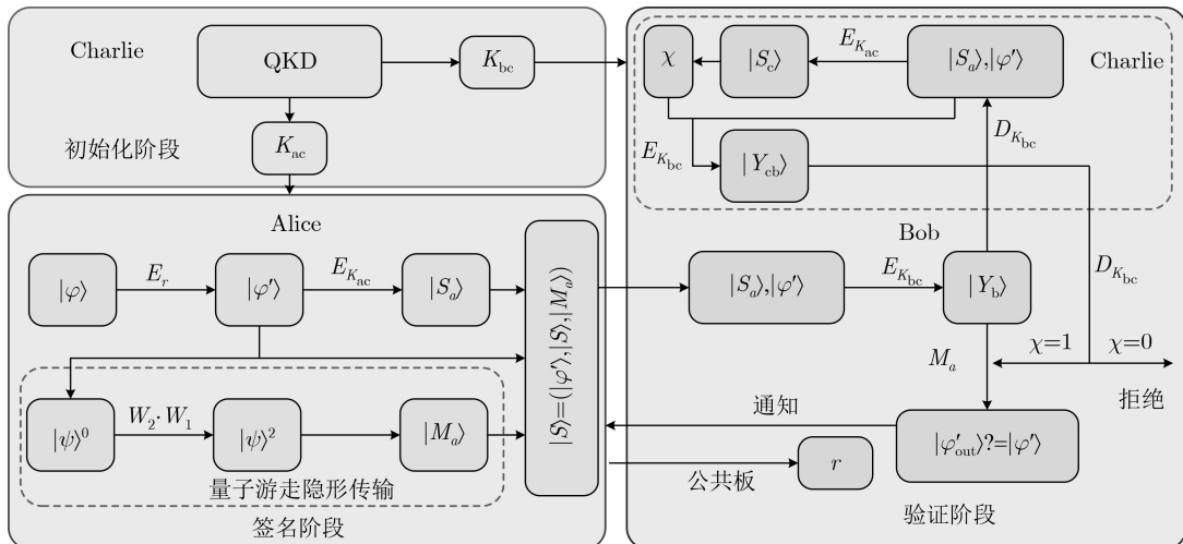
图4 基于 d 正则图量子游走的AQS算法的原理图
