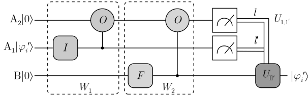
图2 基于两个硬币量子游走的隐形传输线路原理图
