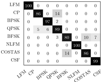
图6 基于小波脊频级联特征识别结果的混淆矩阵
