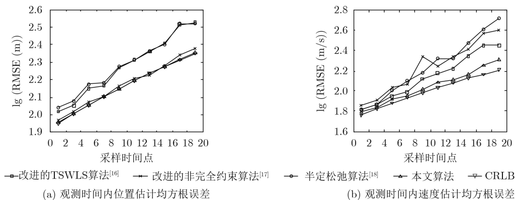
图3 不同时刻目标估计均方根误差对比
