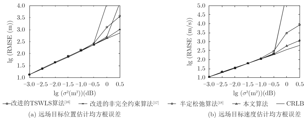
图2 远场目标估计均方根误差对比
