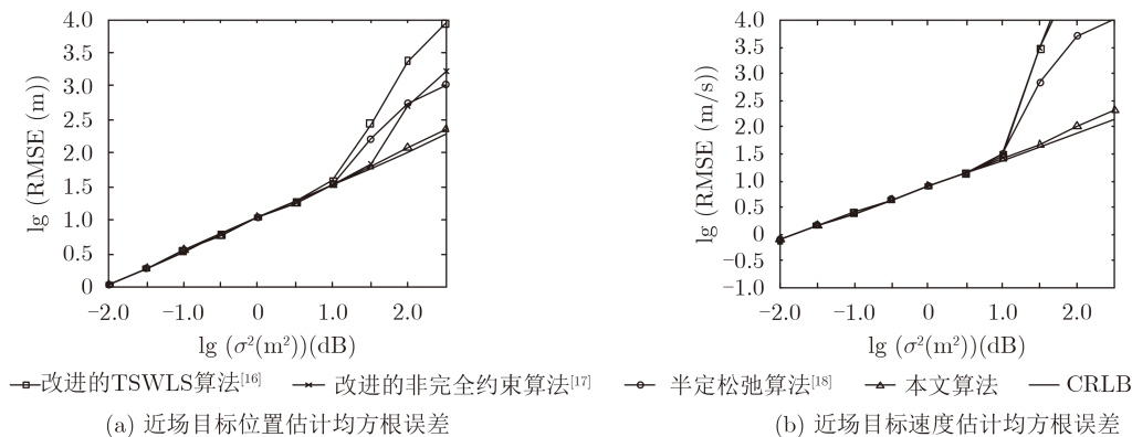
图1 近场目标估计均方根误差对比
