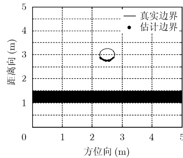
图 11 收发分置下穿墙目标边界成像
