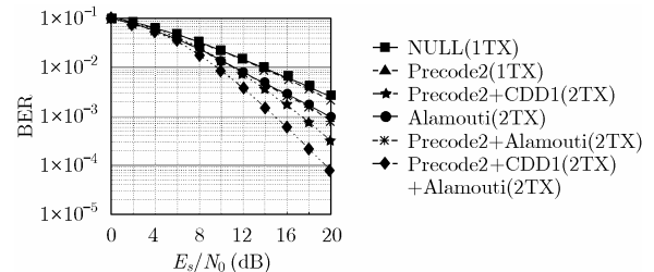
图 5 采用不同编码方式下模型 C 的误比特率曲线
