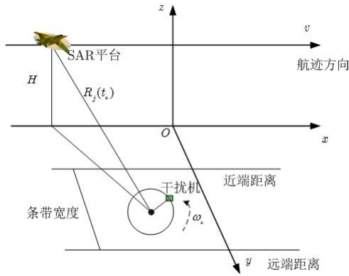
图 1 干扰示意图
