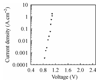
图 4 正向电流-电压特性
