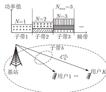
图1 下行NOMA的系统模型
