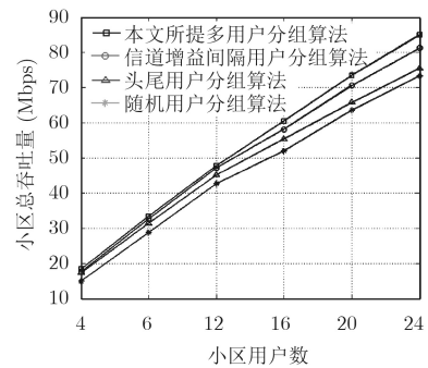
图5 小区用户数与总吞吐量的关系( N=2 )
