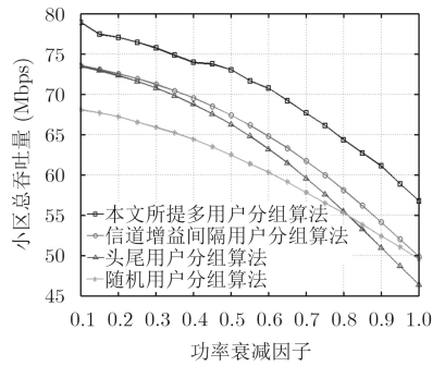
图3 功率衰减因子与总吞吐量的关系( N=3 )
