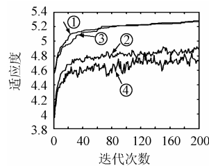
① 免疫进化算法最大适应度 ② 免疫进化算法平均适应度 ③ 进化算法最大适应度 ④ 进化算法平均适应度
