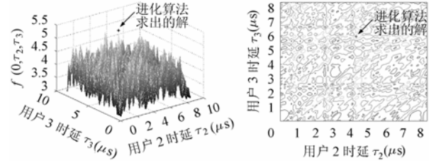
图 2 函数值曲线
