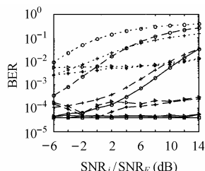
图 8 信干比与误码率
