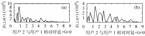
图 1 用户 2 与用户 1 部分互相关函数绝对值与相对时延 \tau 的 PDF 乘积
