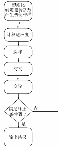
图 4 求解最强和最弱 MAI 条件进化算法框图
