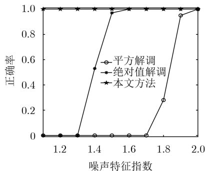
图7 噪声特征指数对叶频估计性能影响
