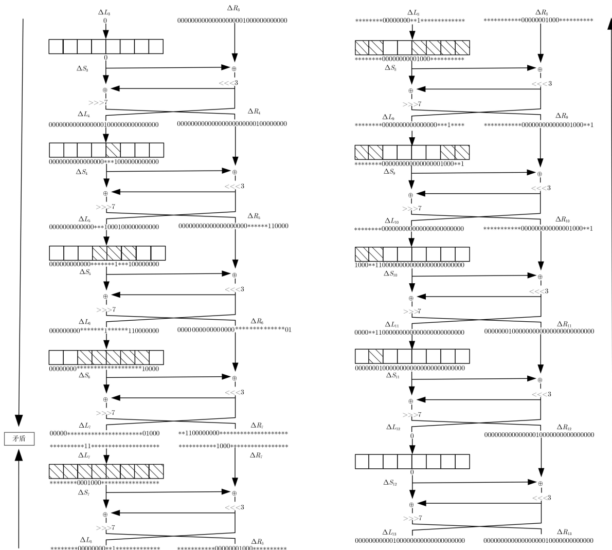
图 2 LiCi算法的10轮不可能差分路线
