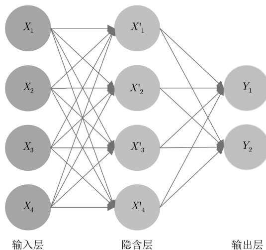
图3 神经网络架构
