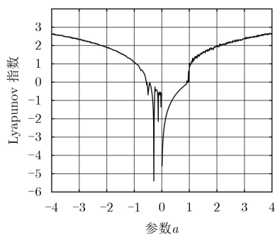
图4 系统式(16)的Lyapunov指数谱
