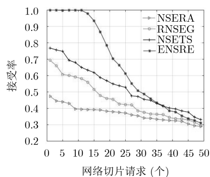
图4 不同算法NSR平均接受率比较
