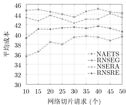
图2 不同算法平均成本比较
