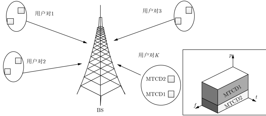
图1 非正交多址K个用户对系统模型
