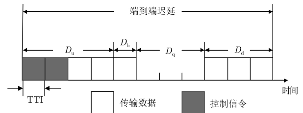
图2 短帧结构
