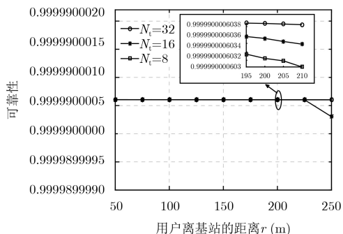
图3 用户离基站的距离与可靠性的关系曲线
