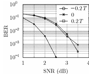
图 3 符号同步误差对 LDPC 译码性能的影响
