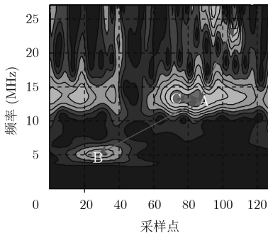
图 3 仿真信号S变换2维时频等高图
