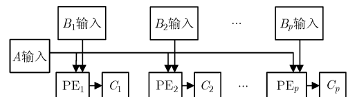
图 10 矩阵乘法器结构示意图
