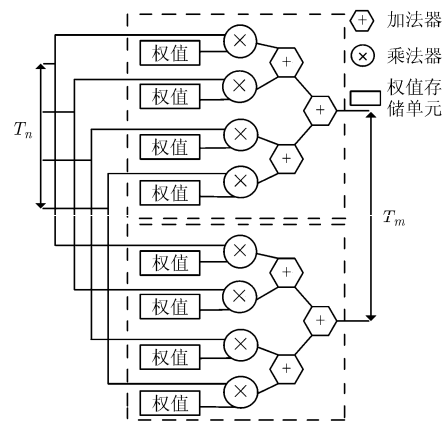
图11 文献[9]卷积计算单元硬件结构
