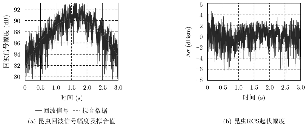
图6 昆虫RCS起伏
