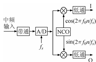
图1 直接中频采样数字正交接收机原理图
