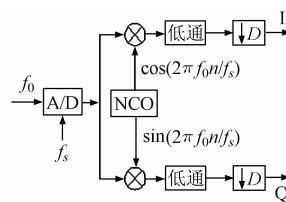
图2 含抽取正交解调的直接实现形式
