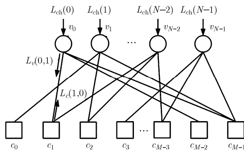
图1 Tanner 图与 BP 译码算法
