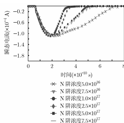
图 14 从 PMOS( P_1 )漏端电流
