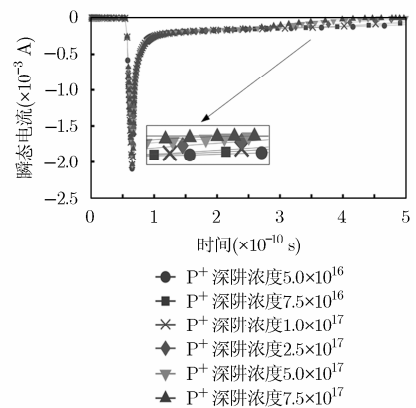
图 9 主 PMOS ( P_0 ) 漏端电流
