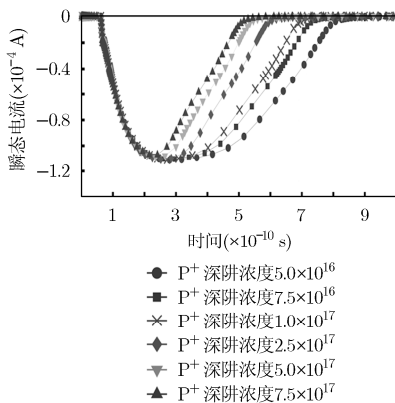
图 10 从 PMOS ( P_1 ) 漏端电流
