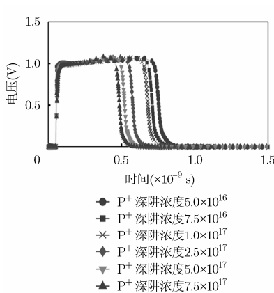
图 7 入射粒子线性能量传输值为 25 \text{ MeV} \cdot \text{cm}^2/\text{mg} , 不同 P + 深阱掺杂下的 Q 点的电压波形的比较
