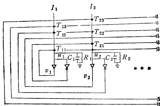
图 1 Hopfield 神经网络模型
