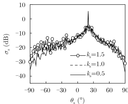
图9 目标尺度对复合散射系数的影响
