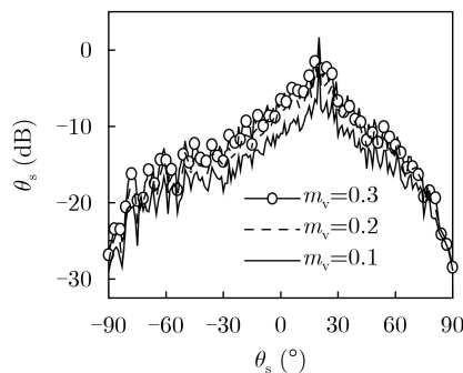
图8 土壤湿度对复合散射系数的影响
