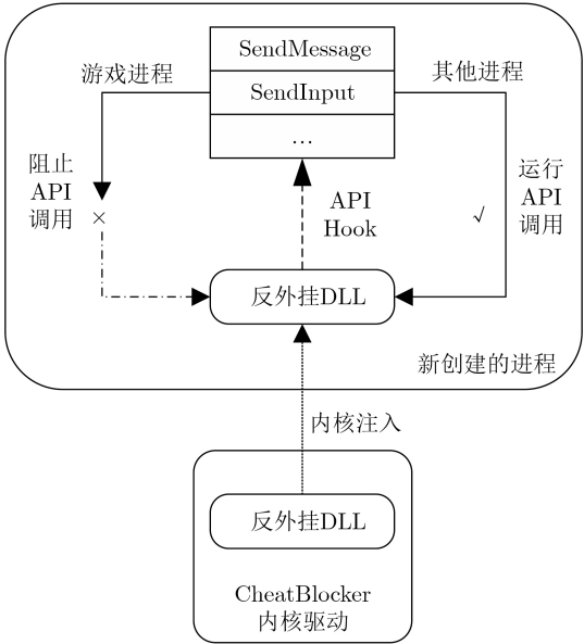
图 5 防御用户输入模拟
