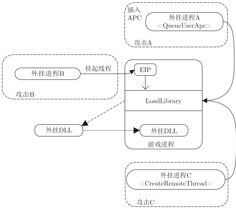
图1 基于跨进程访问的注入方法
