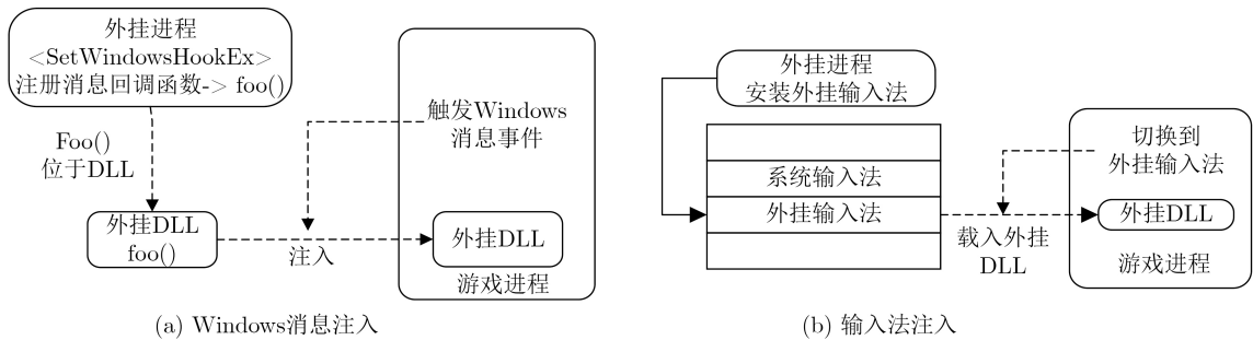
图2 基于系统机制的注入方法
