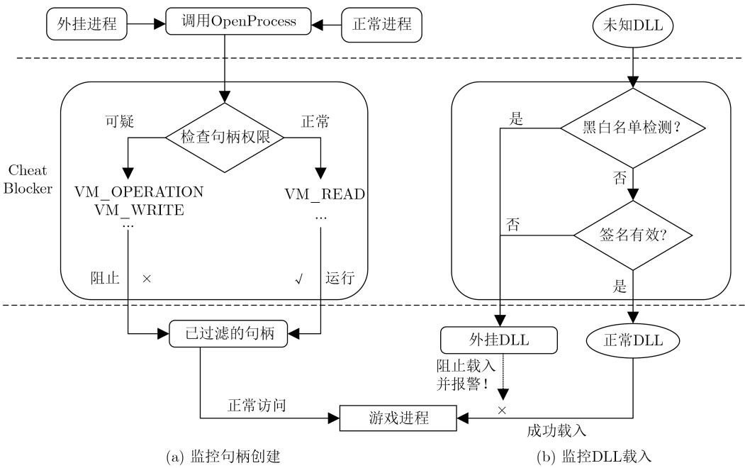
图 4 模块注入防御
