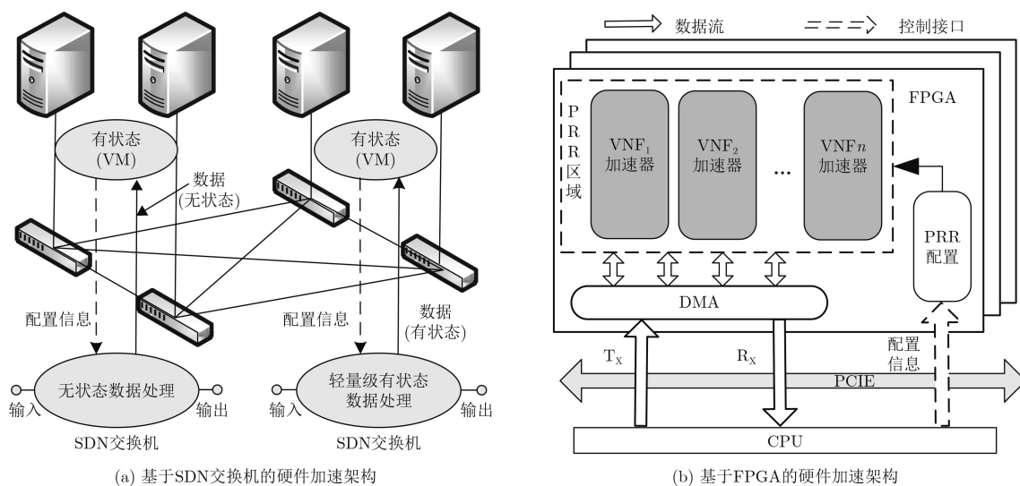
图1 硬件加速资源对网络功能的承载
