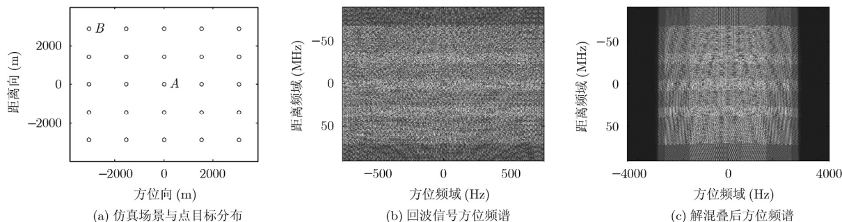
图 6 仿真结果
