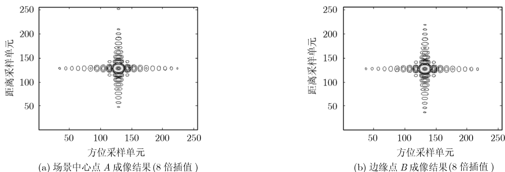
图 7 场景中心 A 和边缘点 B 成像结果
