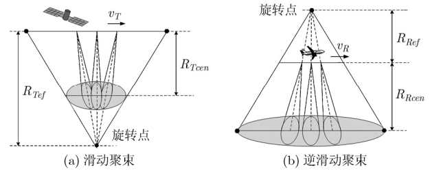
图2 滑动聚束/逆滑动聚束示意图
