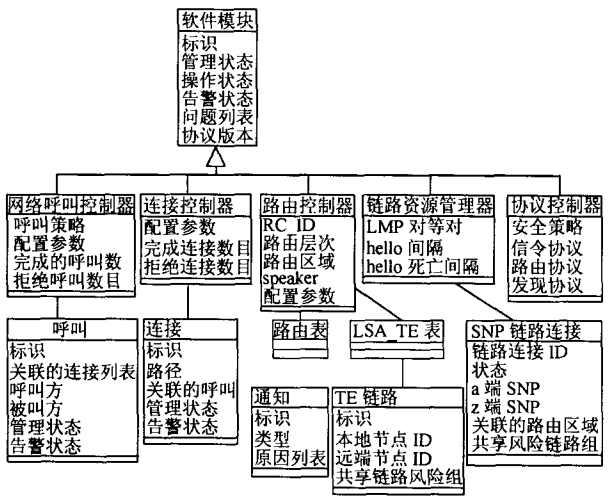
图 5 ASON 控制模块资源对象模型设计
