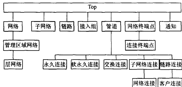
图 1 网络层对象类的包容关系
