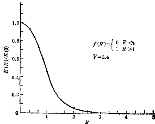
图2 梯度光纤的近场分布
