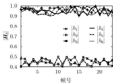
图5 第2种目标RCS模型
