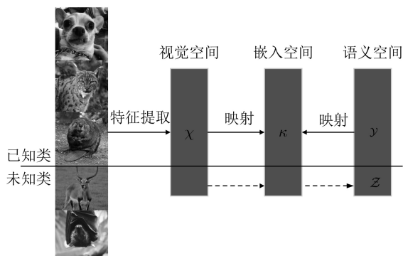
图1 零样本学习技术结构图
