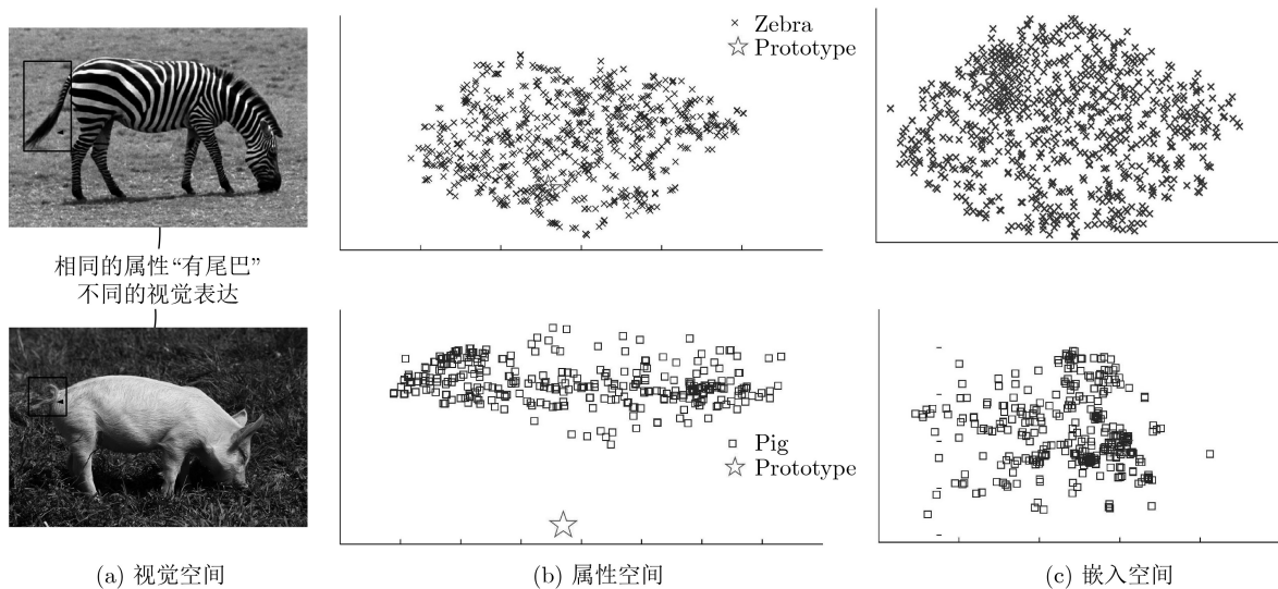
图6 领域漂移示例图 [55]
