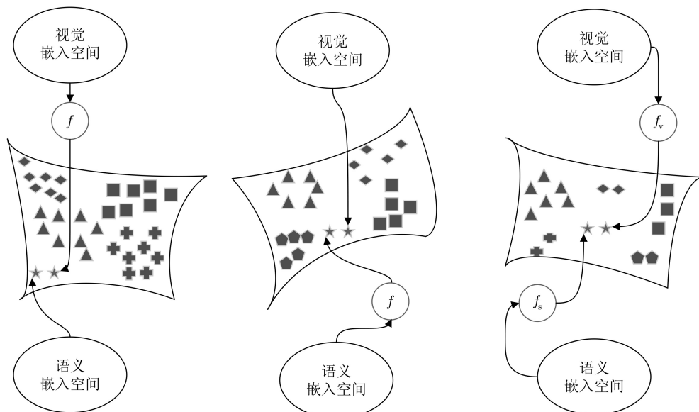
图5 3种视觉-语义映射示意图
