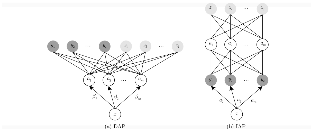
图3 经典归纳式零样本模型示意图 [7]
