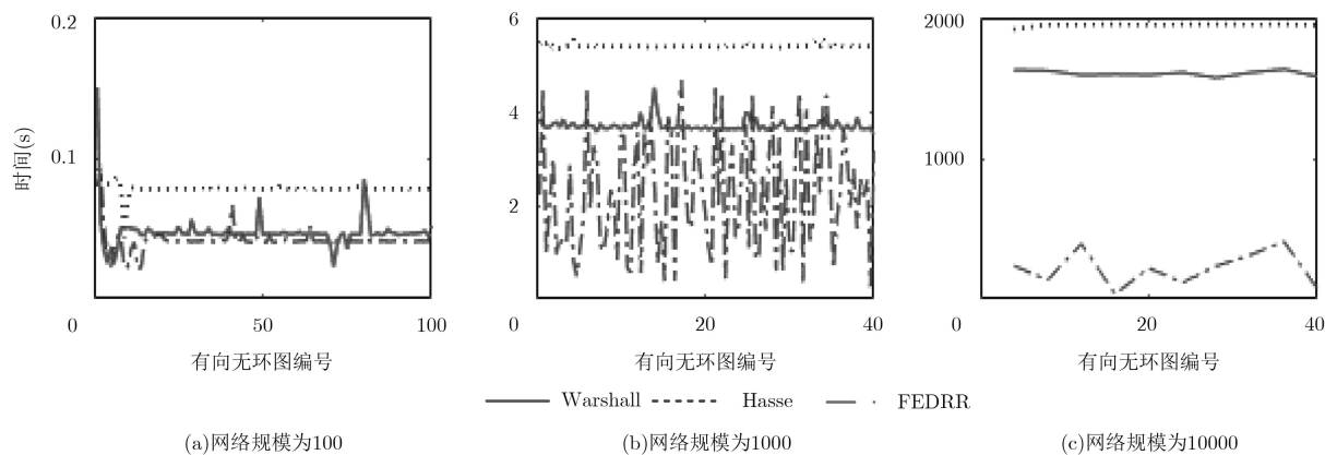
图3 3种算法在不同规模网络下的运行时间
