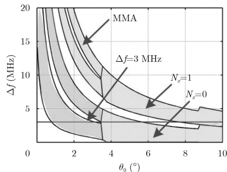
图4 100 km切面多径抑制区
