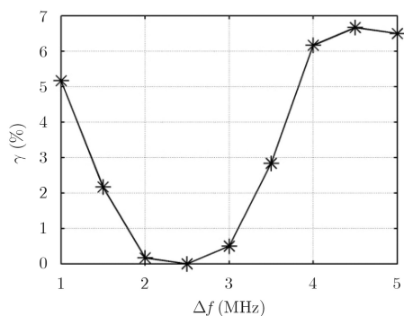
图5 LOR随频偏变化曲线
