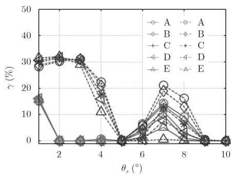
图 7 不同扰动条件下LOR随仰角变化曲线
