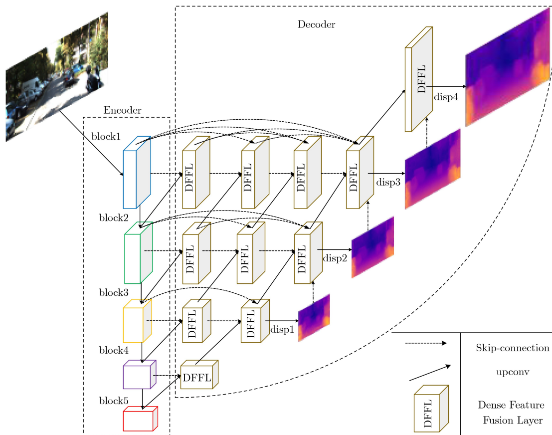
图4 网络框架
