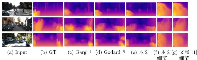
图 5 KITTI数据集上可视化结果对比
